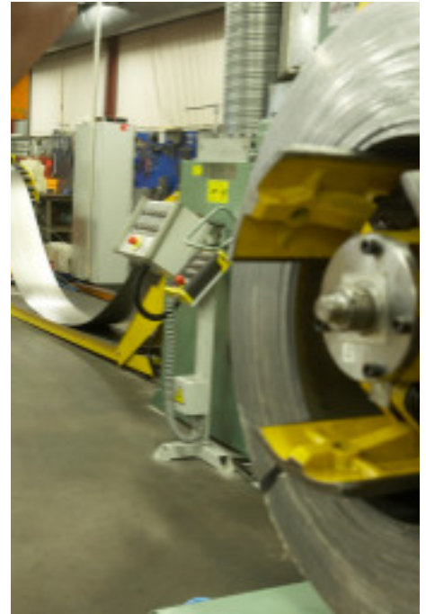
SMV Automatische Presse 1 250 kN mit Bandförderer von Dimeco.
