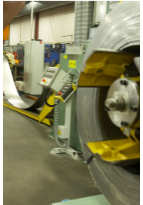
SMV Automatpress 1 250 kN med bandmatning från Dimeco.
